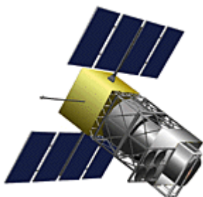
Satélite artificial.
