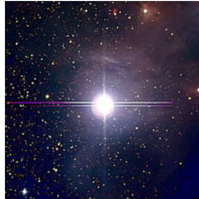
Estrellas
