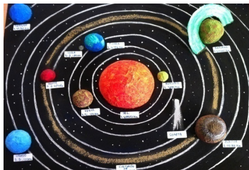
Los planetas
